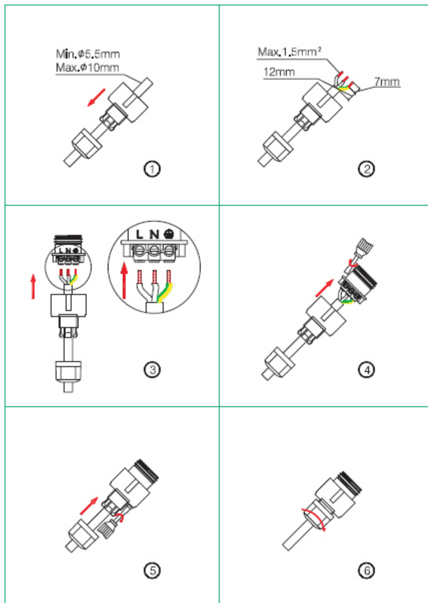
Verbindung des Pumpenanschlusskabels zum externen Netzschalter
