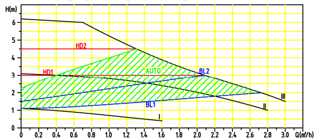
LPA 25-6m Kennlinie
