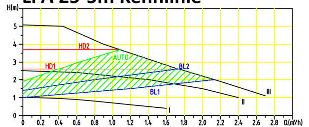
LPA 25-5m Kennlinie
