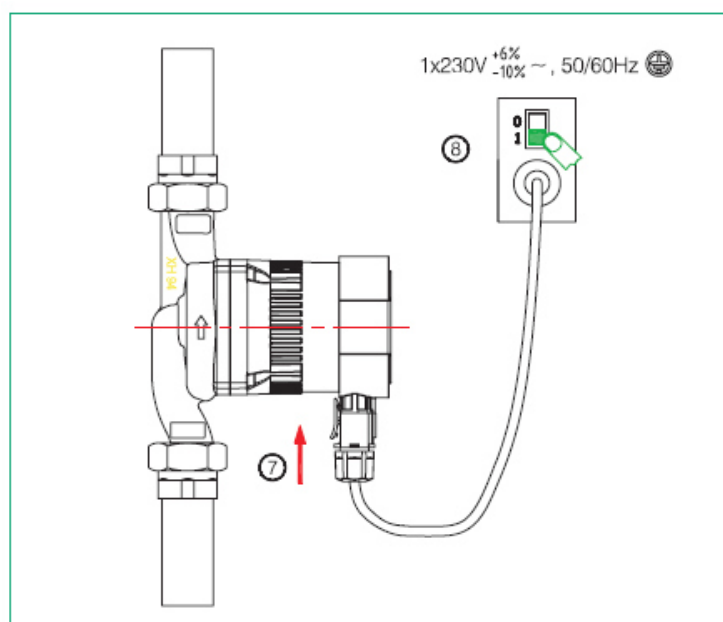
Verbindung des Pumpenanschlusskabels zum externen Netzschalter
