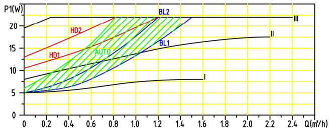
LPA 25-6m Kennlinie
