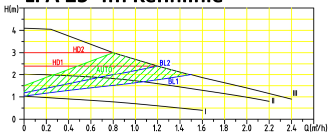
LPA 25-4m Kennlinie
